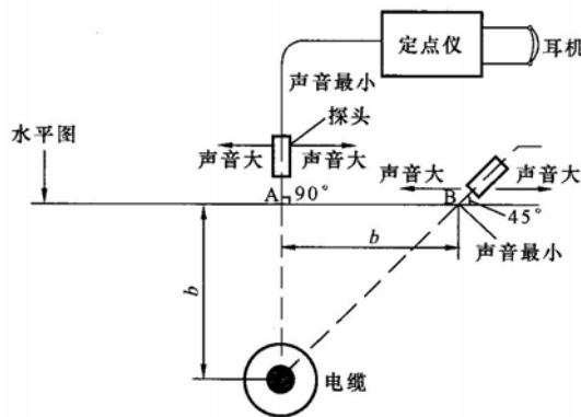
图 2 寻找电缆路径、埋入深度示意图
