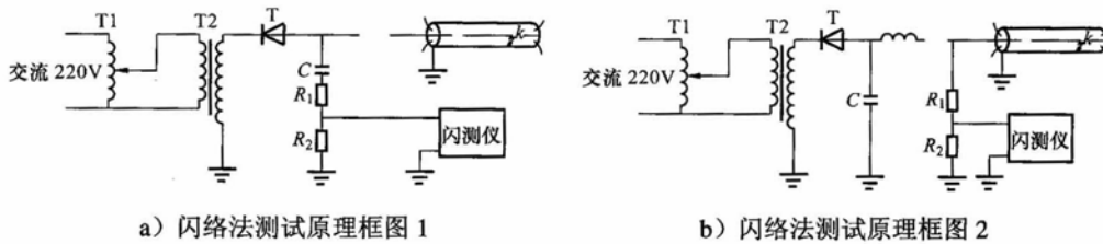
图 2 闪络法测试原理框图
