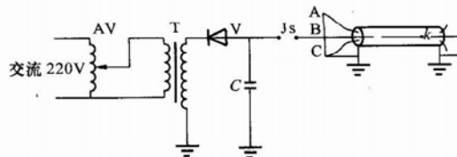
图 2 开路故障定点测试连接线路
