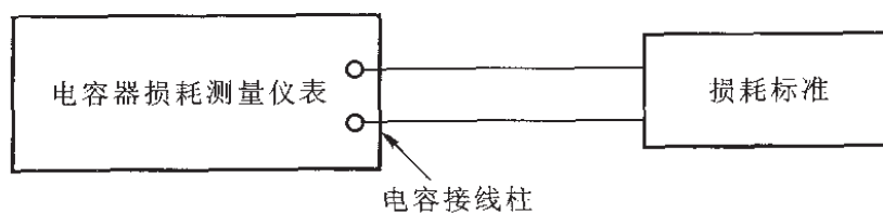
图2 损耗值的校准连接
